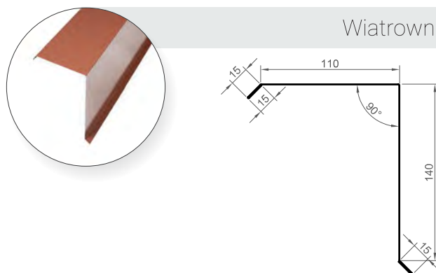
Wiatrownica GRANDE
