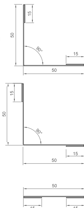
Narożnik wewnętrzny
